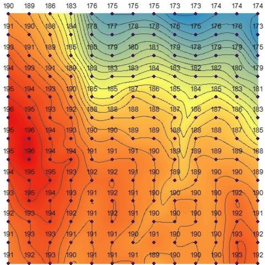
ภาพที่ 9 ค่าความสูงจากระดับน้ำทะเลปานกลาง (เมตร) ของแต่ละหมุดย่อย
